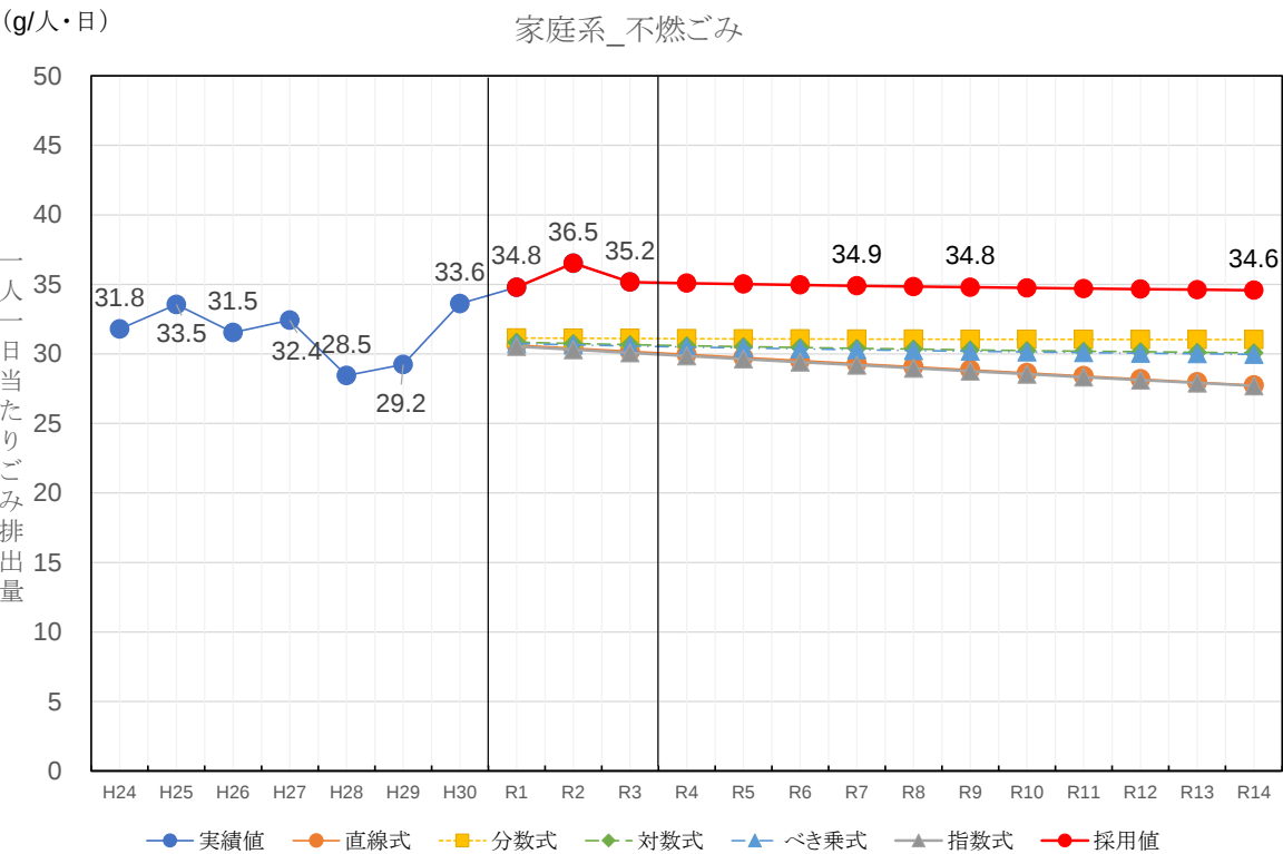
図 7-2 北秋田市における家庭系不燃ごみ量原単位の各推計式による推計結果
