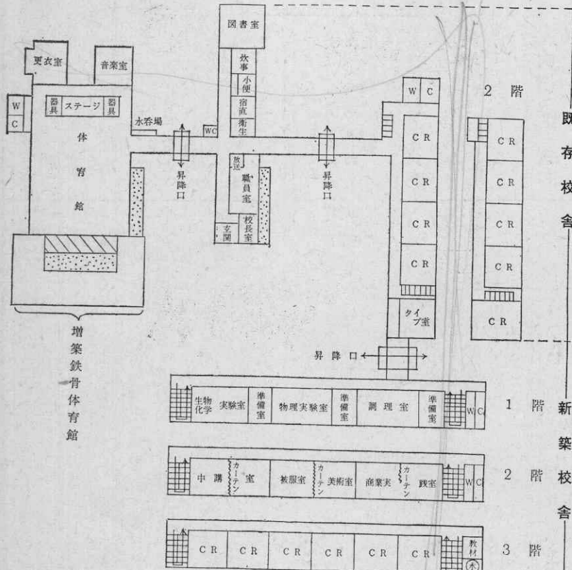
配置図
