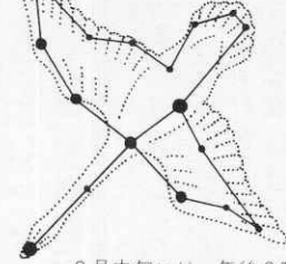
8月中旬には、午後9時ごろ頭の上(天頂)に見えます
