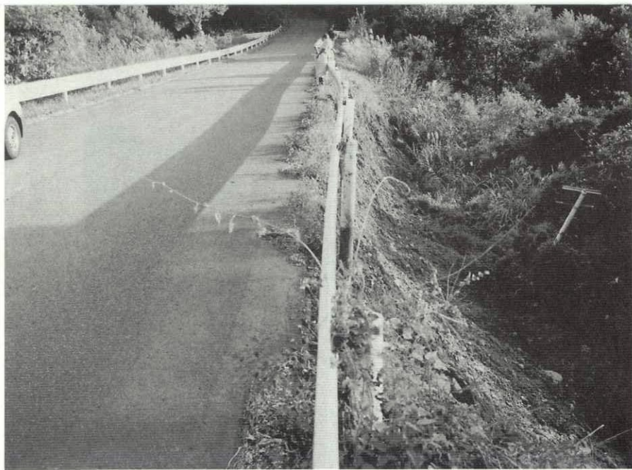
8月25日の集中豪雨で、一部が崩壊した町道大野台中央線
