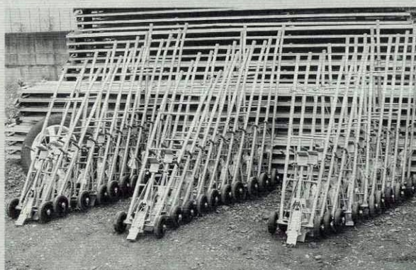
←道路側溝コンクリート蓋脱着機
