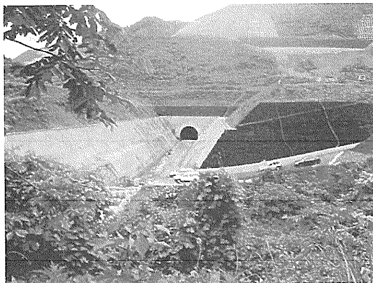
貫通した森吉山ダム下段仮排水路トンネル全景 (呑口側より撮影 平成12年6月)
