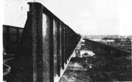
米代川堤防かさあげによる阿仁合線 薩摩・小ヶ田間の新鉄橋―左側
