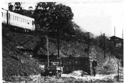
昨年9月着工した坊沢～大野尻間の農免道路は本年度中に完成する —米代川に架けられる橋りょう工事—
