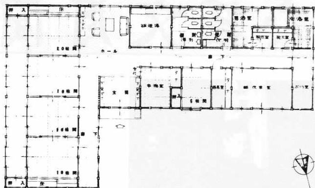
老人いこいの家平面図
