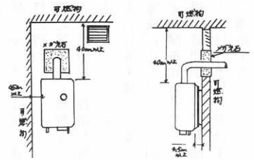
「簡易給湯器（入力10,000キロカロリー以下）は図のように取り付けてください。」
