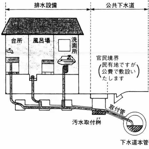
排水設備図（例）
