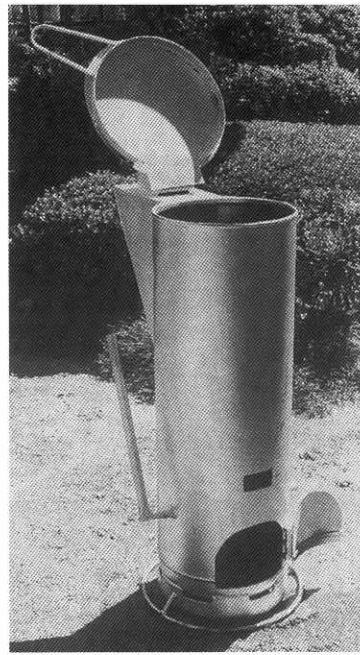
ガスボンベ改良型焼却炉
