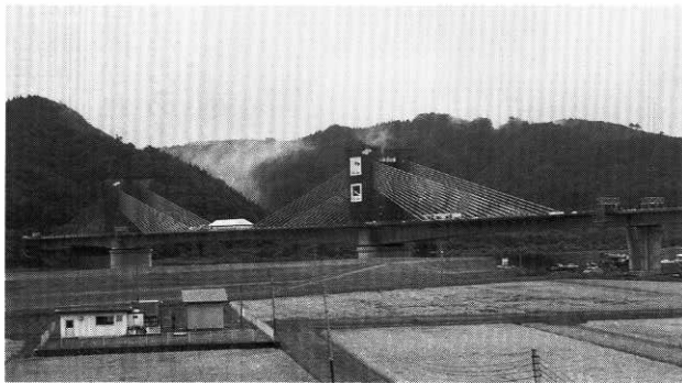
中央部が連結された蟹沢大橋
