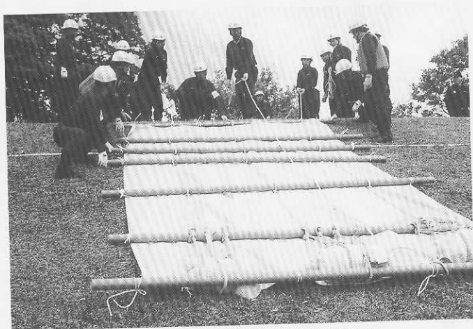
シート張工法の訓練をする水防団員
