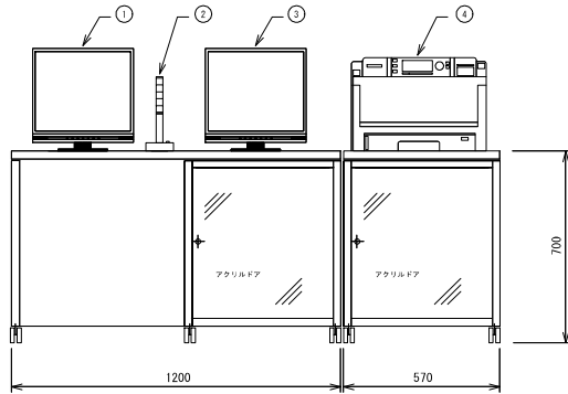
内部配置図
