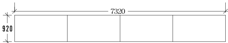
①横看板 W7,320mm×H920mm 板面有り (白塗装)
