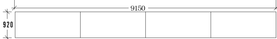
②横看板 W9,150mm×H920mm 板面有り (白塗装)
