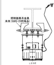
体育館照明器具固定参考図
