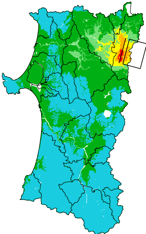
(4) 天長地震
