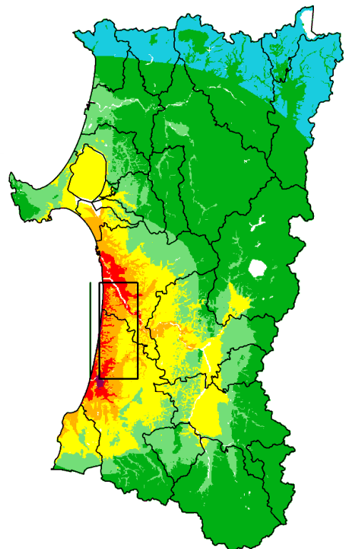
(6) 北由利断層
