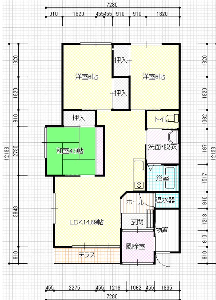
平面図
