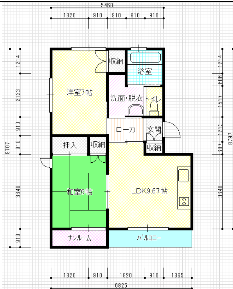
平面図
