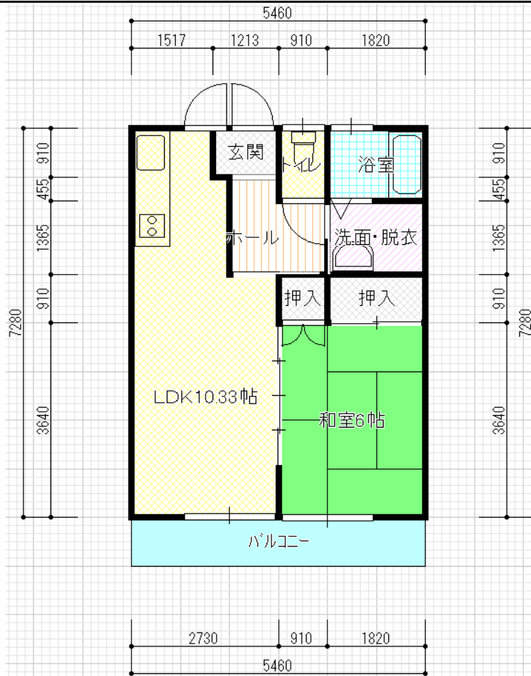
平面図
