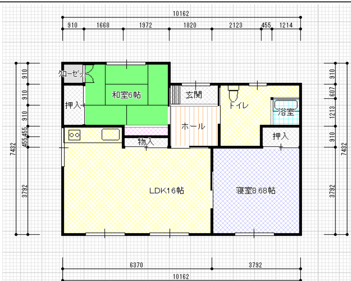
平面図
