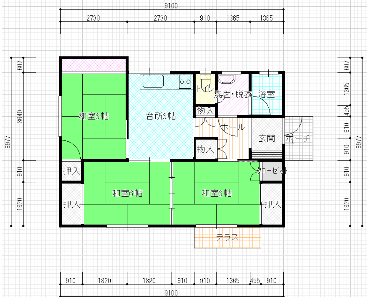
平面図
