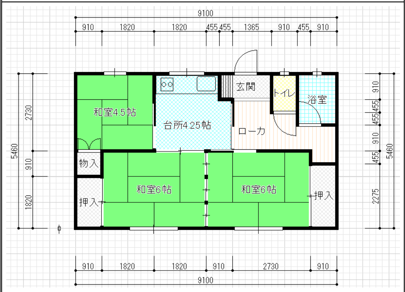
平面図
