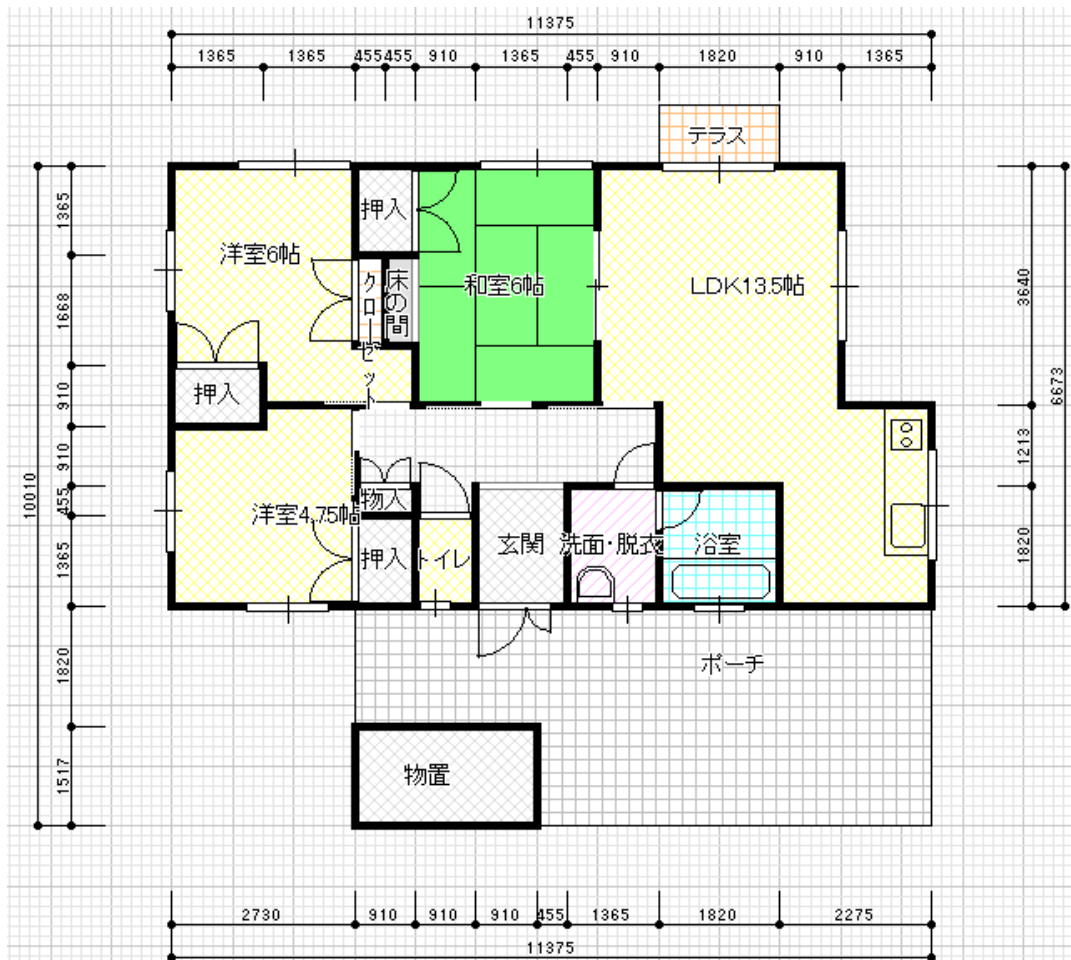
平面図
