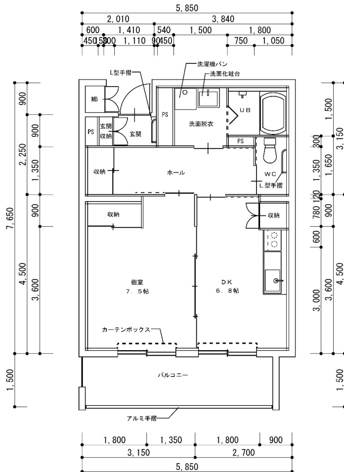
平面図
