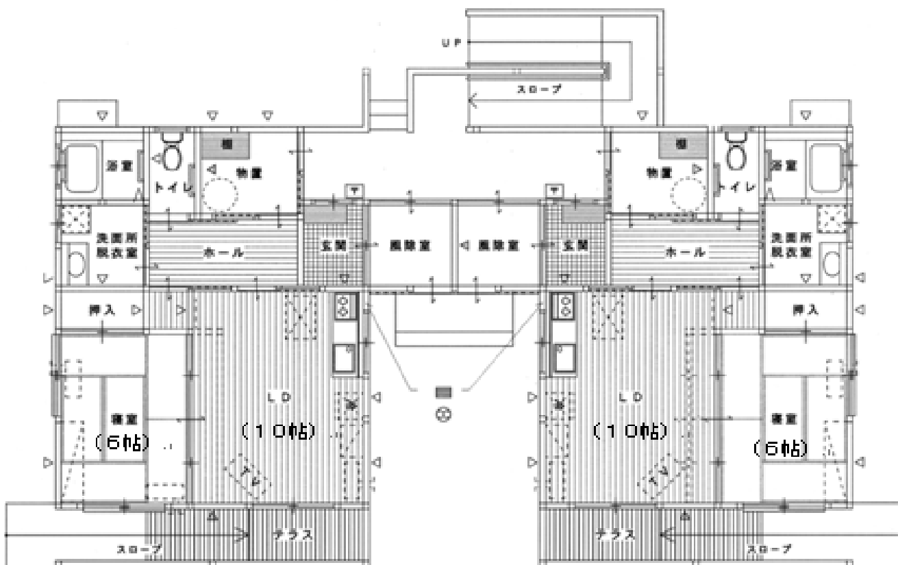
平面図
