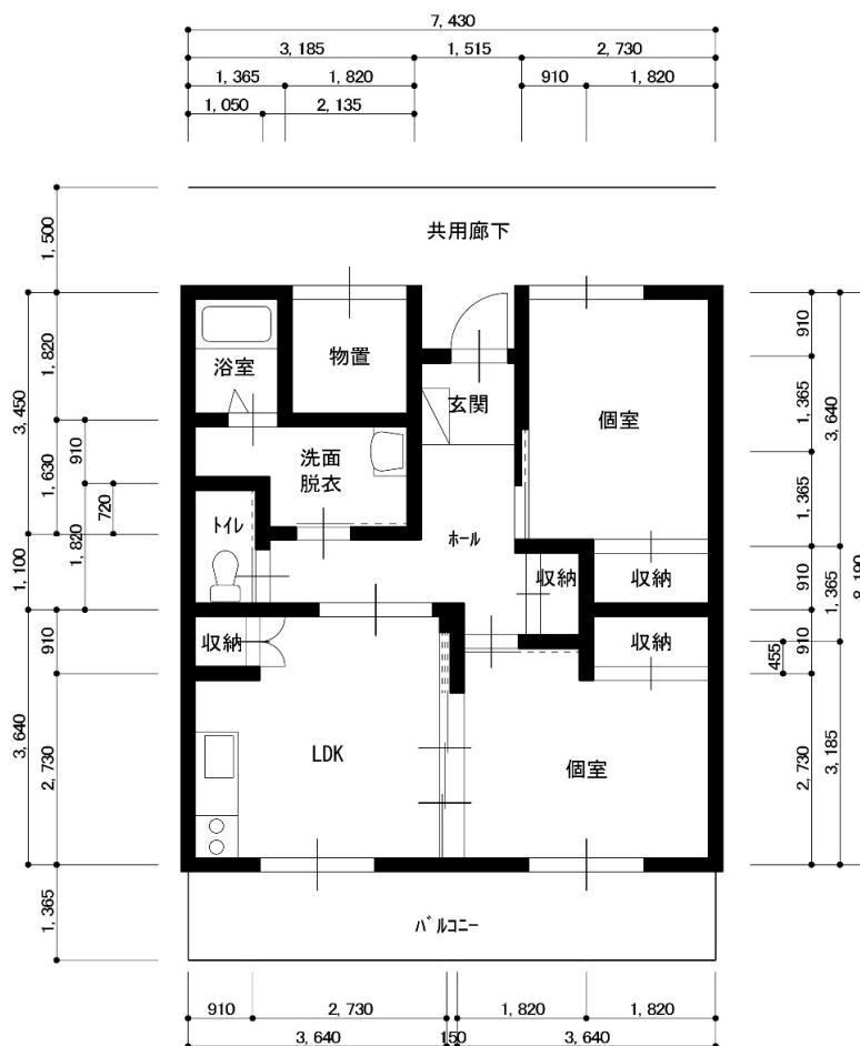
平面図
