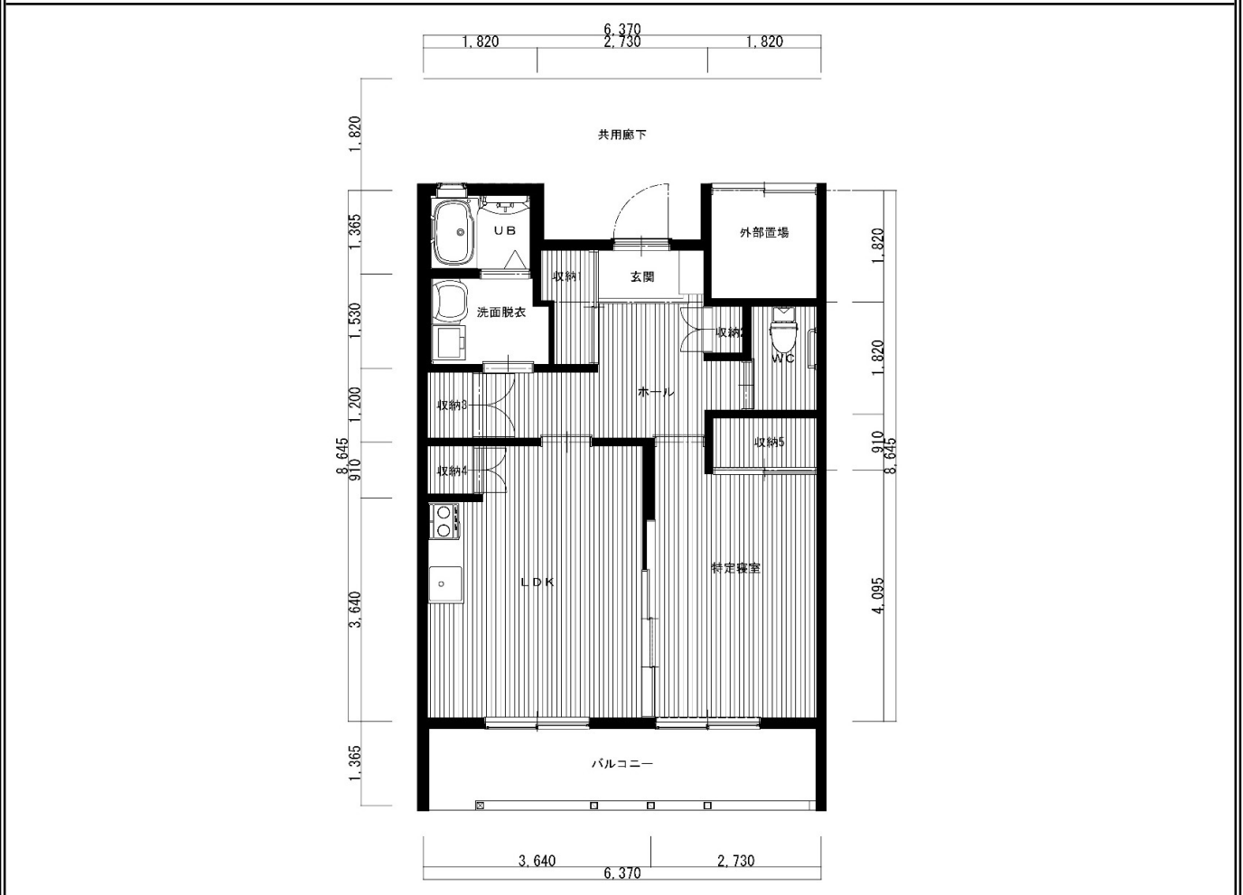
平面図
