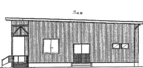
東側 立面図 S:1/100
