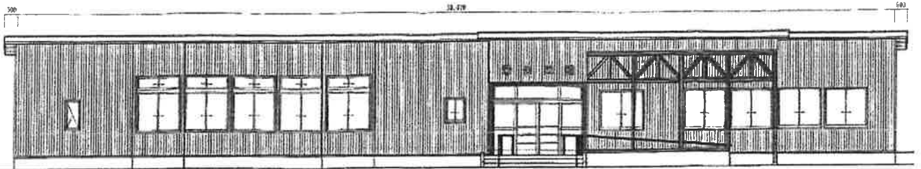
南側 立面図 S:1/100
