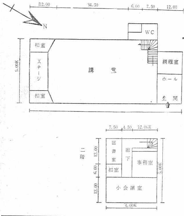
阿仁町吉田公民館見取図 S = 1/200
