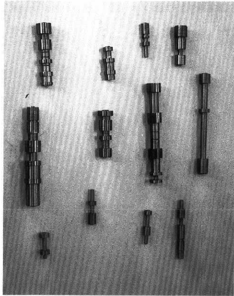
トルコン内部に組み込まれているスプールバルブ
